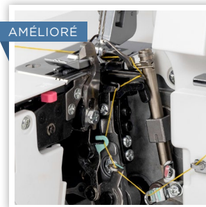
ENFILAGE FACILE DU BOUCLEUR INFÉRIEUR
